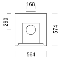
CALOR QUADRA
