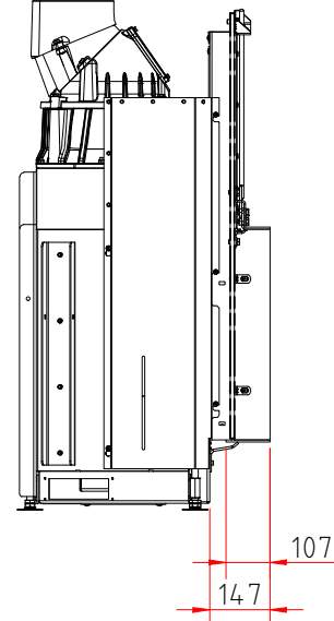
Seitenansicht M 1:20
