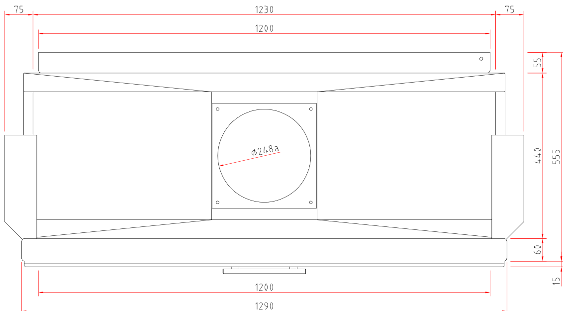
Draufsicht M 1:10
