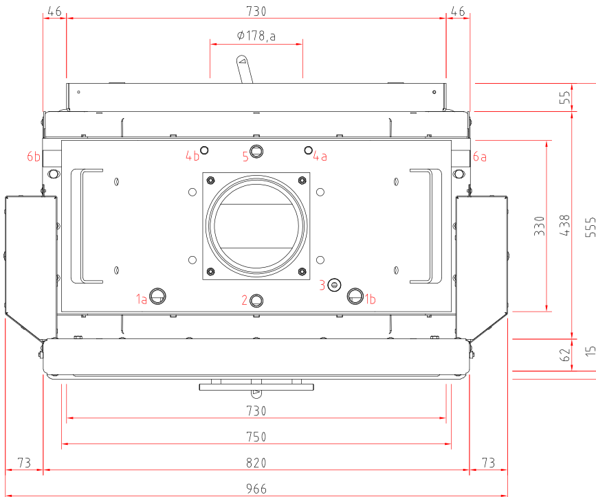
Draufsicht M 1:10
